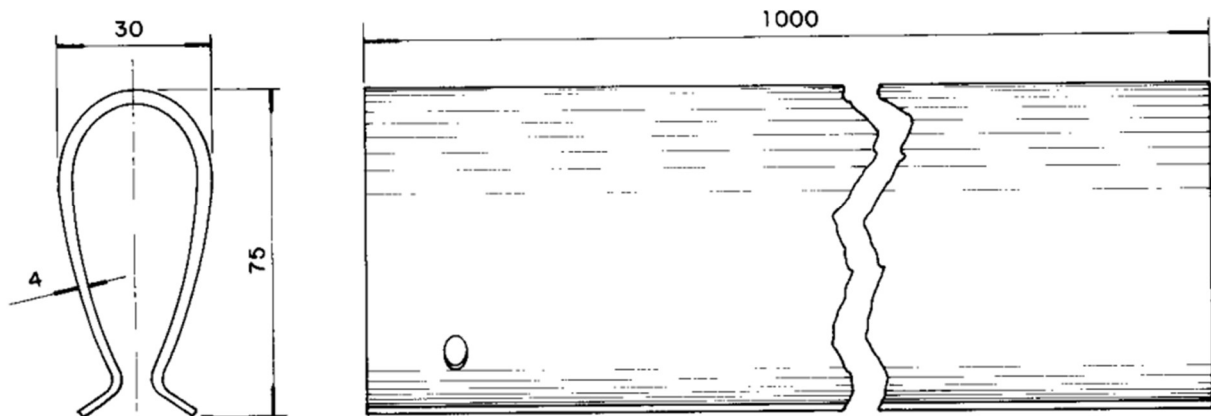
Figura 1 - Calha protetora de Rede Compacta
